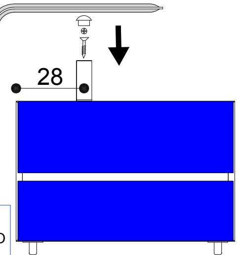
DETALHE - FIXAÇÃO DO ESPAÇADOR COM PARAFUSOS PHILLIPS
