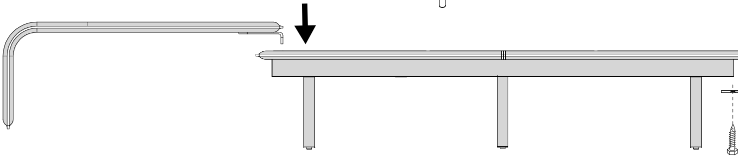
DETALHE - MESA LATERAL L COM ENCAIXE NA PARTE DE CIMA DO ESTRADO
