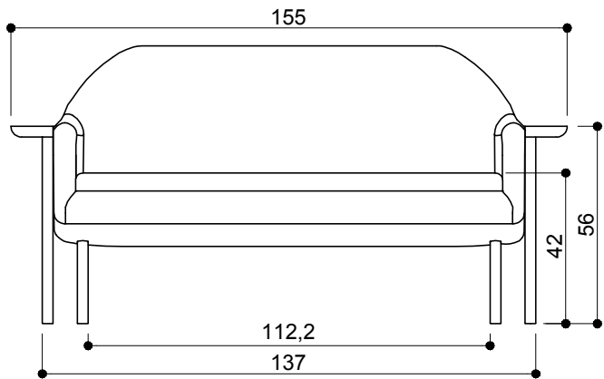
VISTA FRONTAL NAMORADEIRA VOLTA ESCALA 1:1
